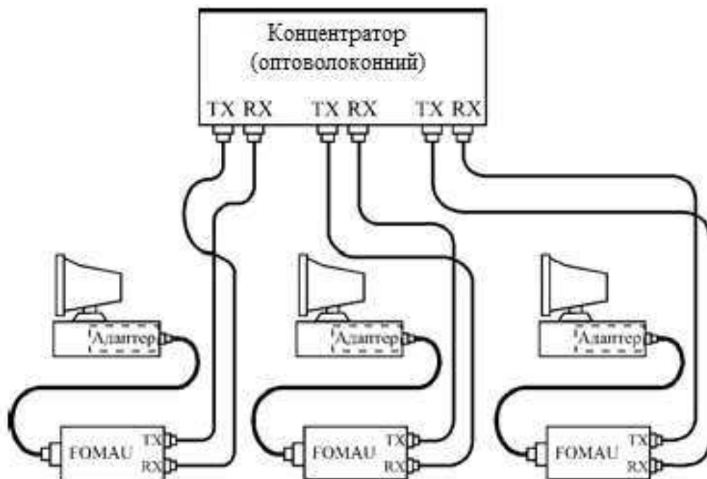
Рисунок 1.15 – Об'єднання комп'ютерів у мережу за стандартом 10BASE-FL
