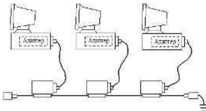
Рисунок 2.3 – Схема з'єднання комп'ютерів сегмента мережі на "товстому" кабелі
