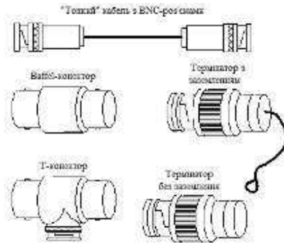
Рисунок 2.4 – Апаратні засоби 10 BASE 2
