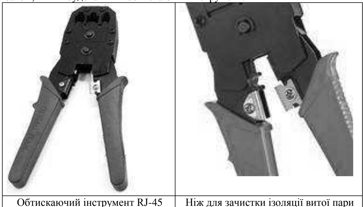
Рисунок 1.23 – Обтискаючий інструмент RJ-45
