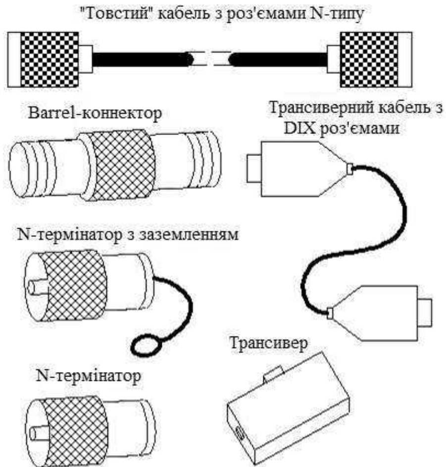
Рисунок 2.2 – Апаратні засоби 10 BASE 5
