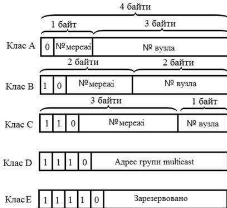
Рисунок 4.4 – Класи адресів
