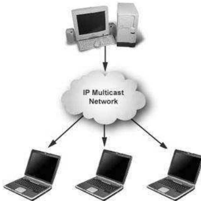
Рисунок 4.4 – Технологія multicast
