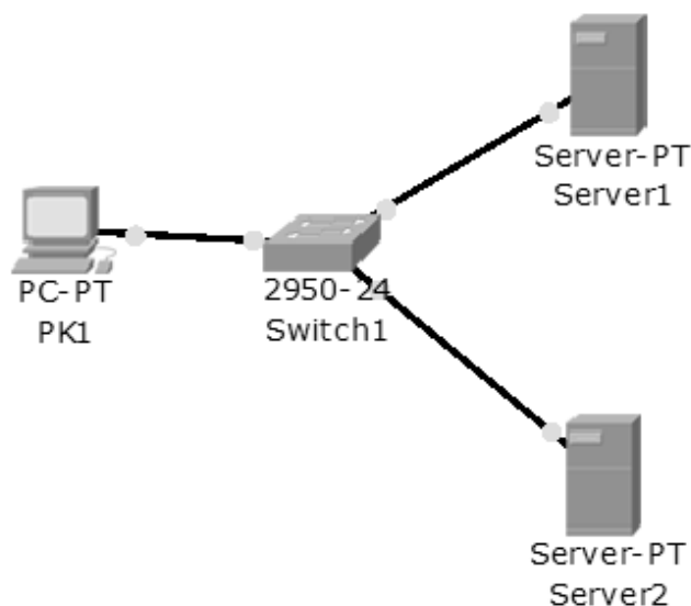
Рисунок 6.1 – Схема мережі
