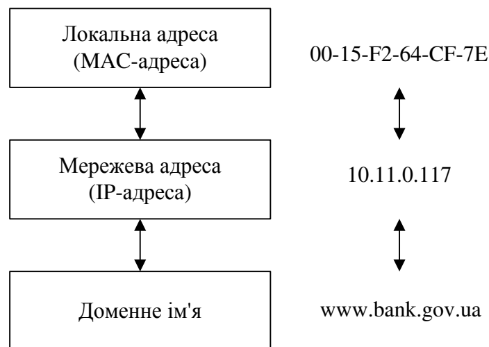
Рисунок 4.2 – Перетворення адрес
