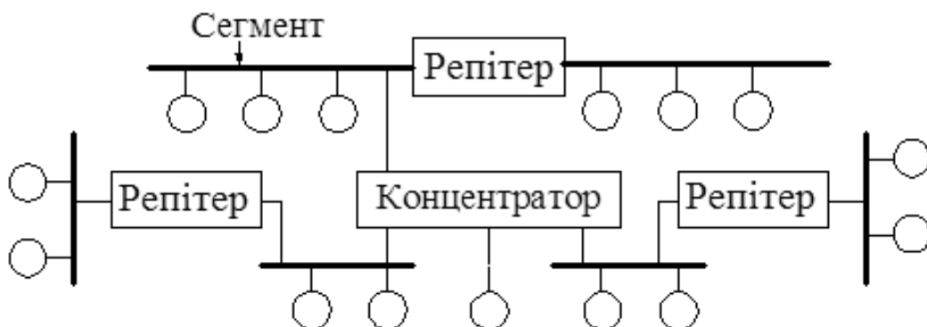
Рисунок 2.1 –Приклад використання репітерів і концентраторів
