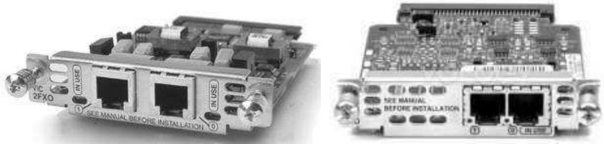
Рисунок 5.9 – Приклади мережевих модулів з голосовим/факс інтерфейсом (VIC2)
