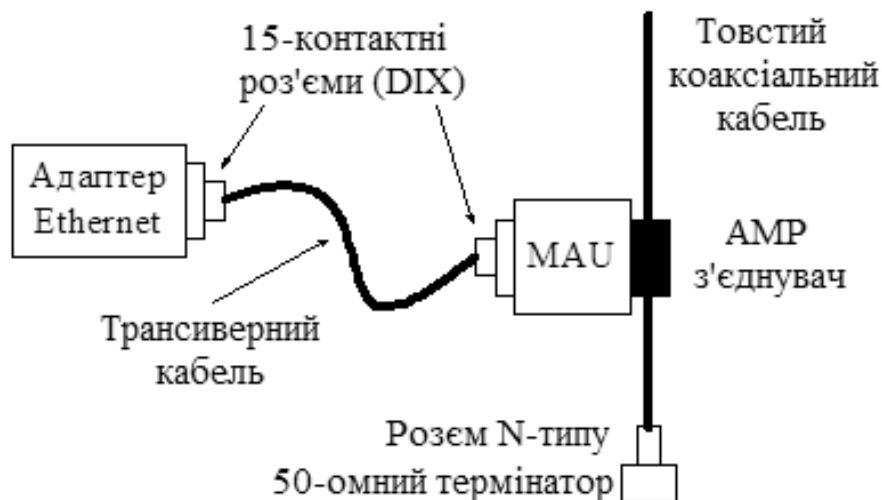
Рисунок 2.3 – Схема під'єднання адаптера до "товстого" кабелю
