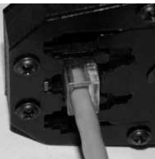
Рисунок 1.29 – Обтискання коннектора з встановленою парою
