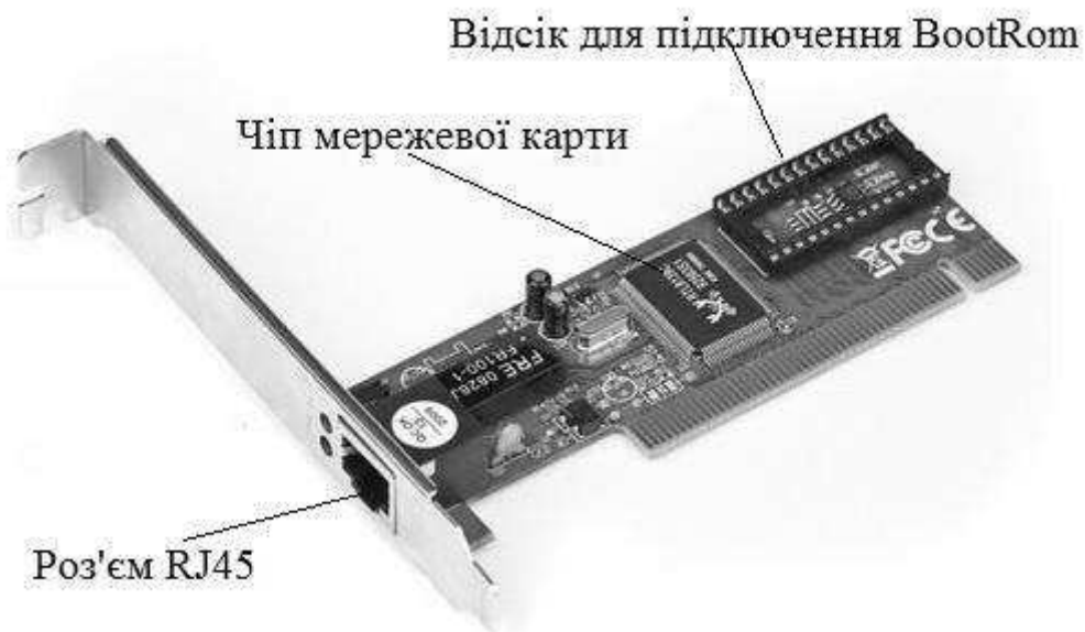
Рисунок 1.1 – Мережева карта
