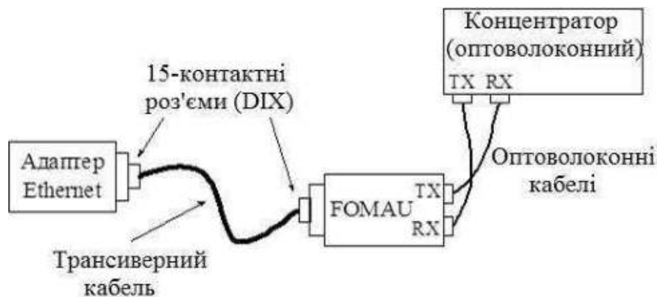
Рисунок 2.6 – Схема з'єднання мережного адаптера і концентратора
