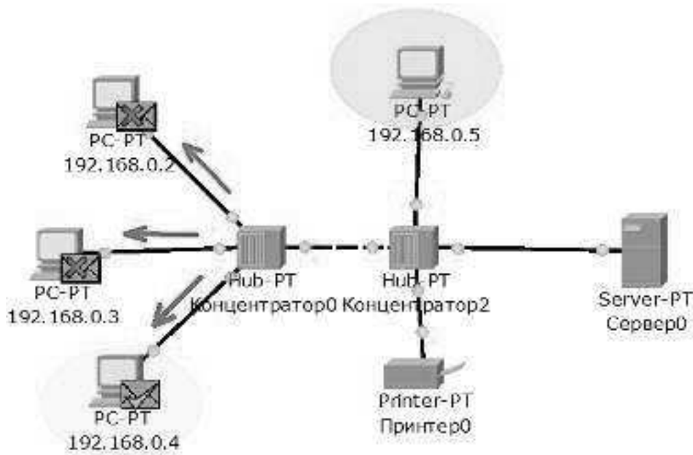
Рисунок 5.31 – Проходження пакету. Кінцевий етап
