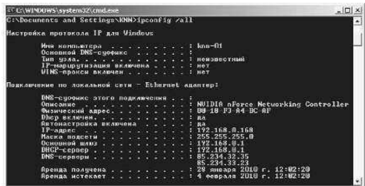
Рисунок 3.1 – Відображення встановлених на комп'ютері мережових конфігурацій утилітою ipconfig
