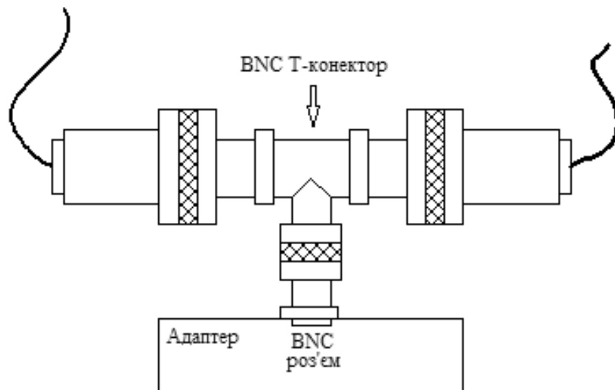
Рисунок 2.5 – Схема під'єднання адаптера по "тонкому" кабелю
