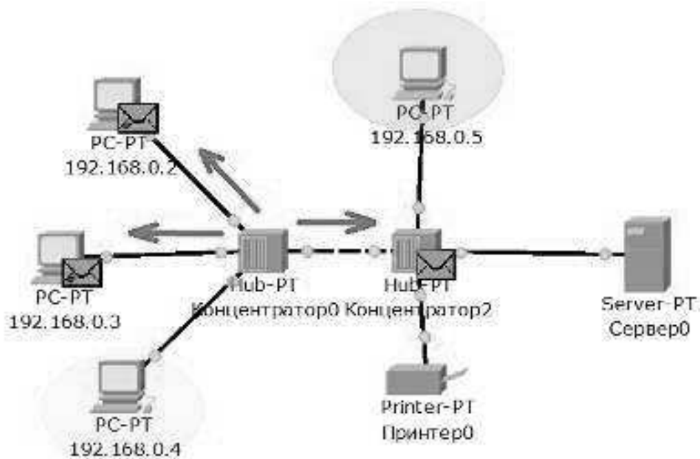
Рисунок 5.27 – Проходження пакету. Другий етап
