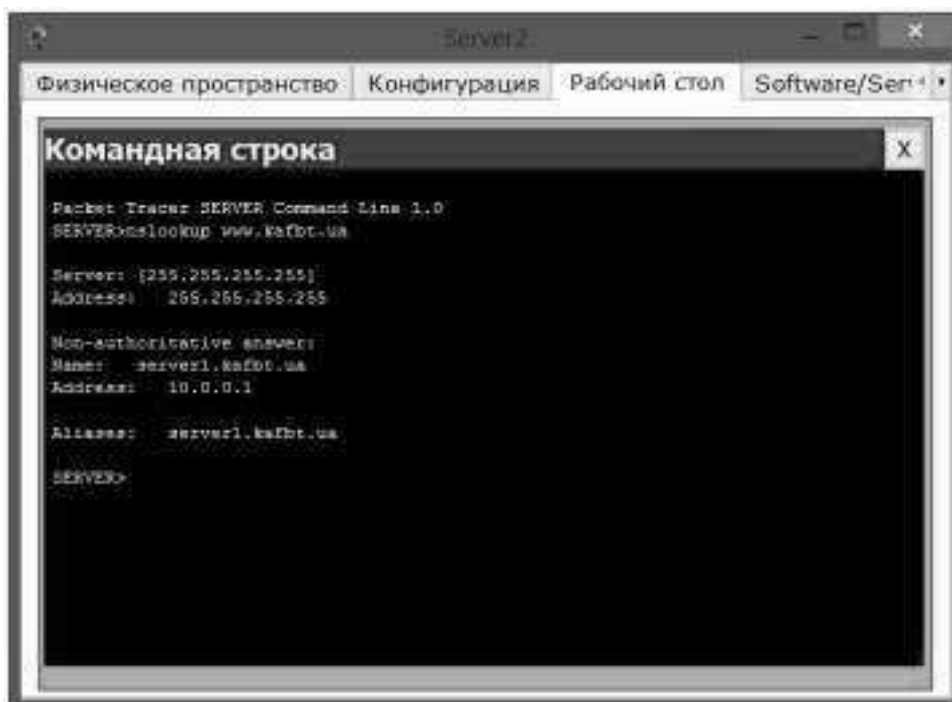
Рисунок 6.7 – Перевірка прямий зони DNS
